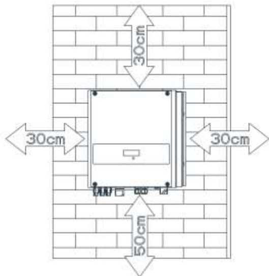
Dimensões ambientais de um inversor
