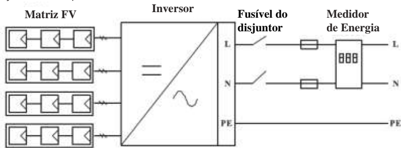
(A) Sistema de inversor único
