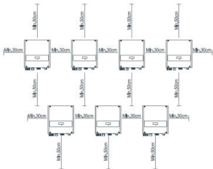
Dimensões ambientais de inversores em série
